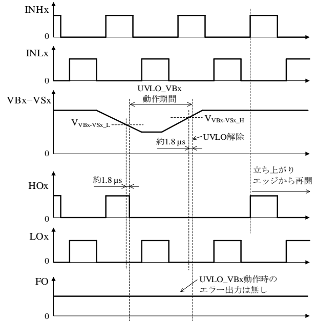
図 13-14 UVLO_VBx 動作波形
