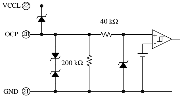
図 8-4 OCP 端子内部回路図
