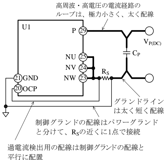
図 14-1 高周波かつ高電圧の電流経路と制御グラウンドの配線
