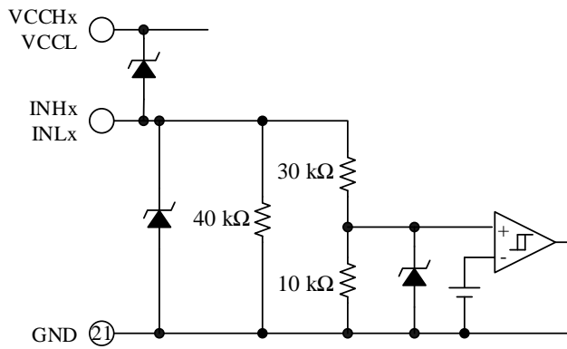
図 8-2 INHx、INLx 端子内部回路図
