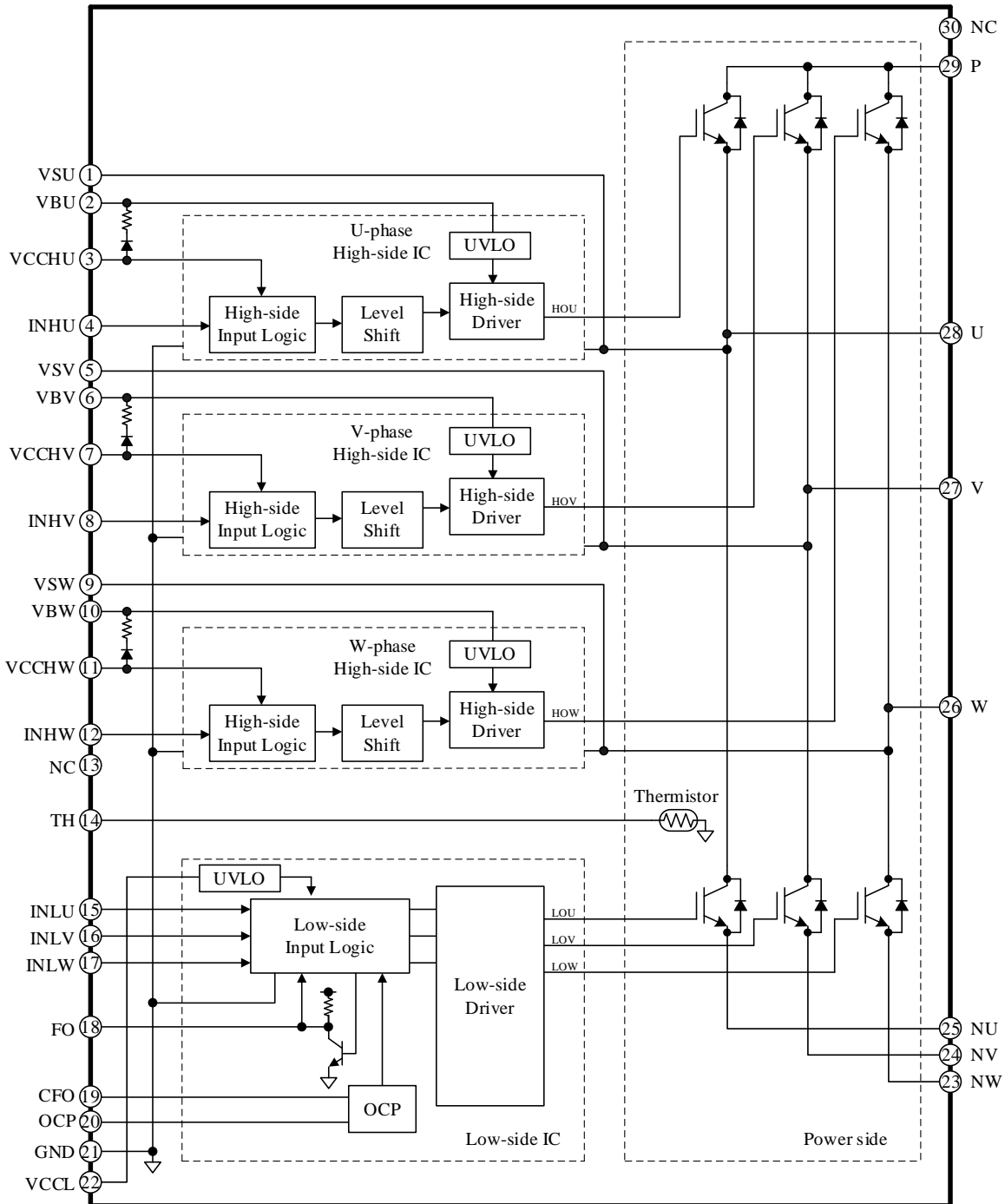
図 8-1 ブロックダイアグラム
