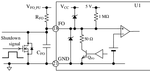
図 13-13 FO 端子の周辺回路と内部回路
