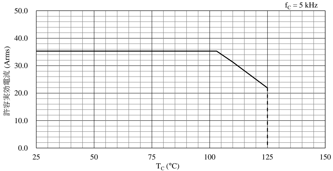
図 16-6 許容電流特性 ( f_C = 5 \text{ kHz} )
