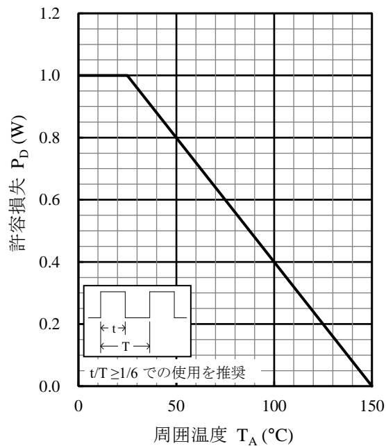
図4 P_D - T_A 特性
