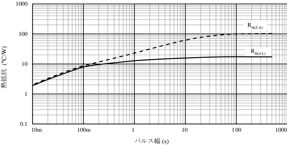
図 9 代表過渡熱抵抗特性
