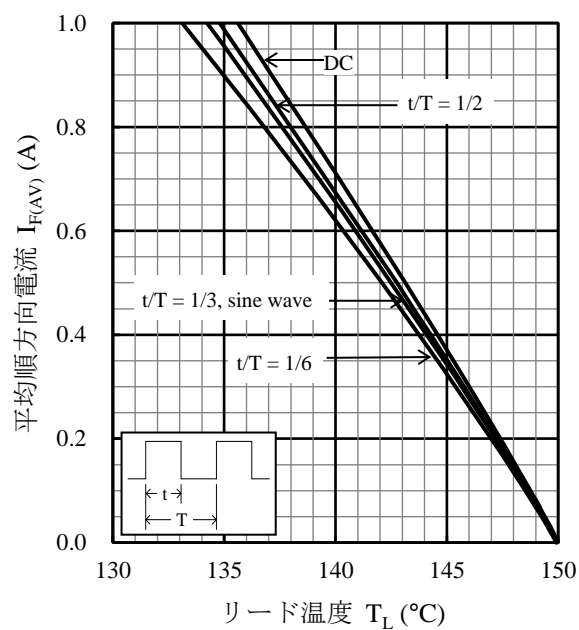
図3 I_{F(AV)} - T_L 特性 ( T_J = 150 °C、 V_R = 100 V)
