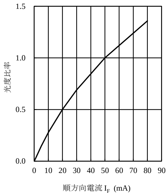
図3 光度比率 - I_F 特性
