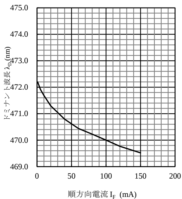
図4 \lambda_D - I_F 特性
