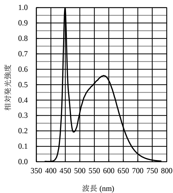
図6 発光スペクトル分布
