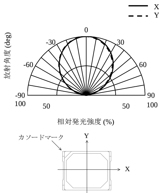
図7 指向性
