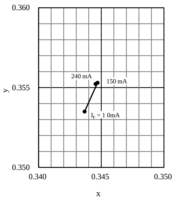
図5 I_F - 色度特性
