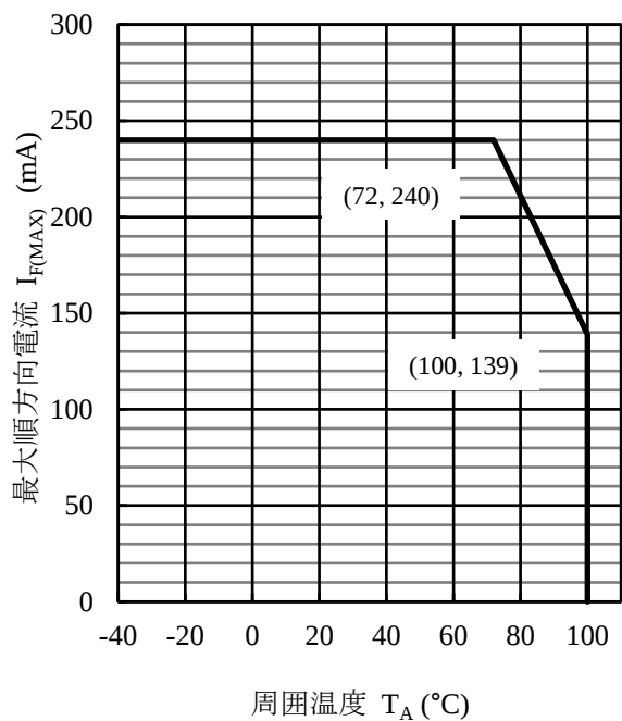
図2 I_{F(MAX)} - T_A 特性
