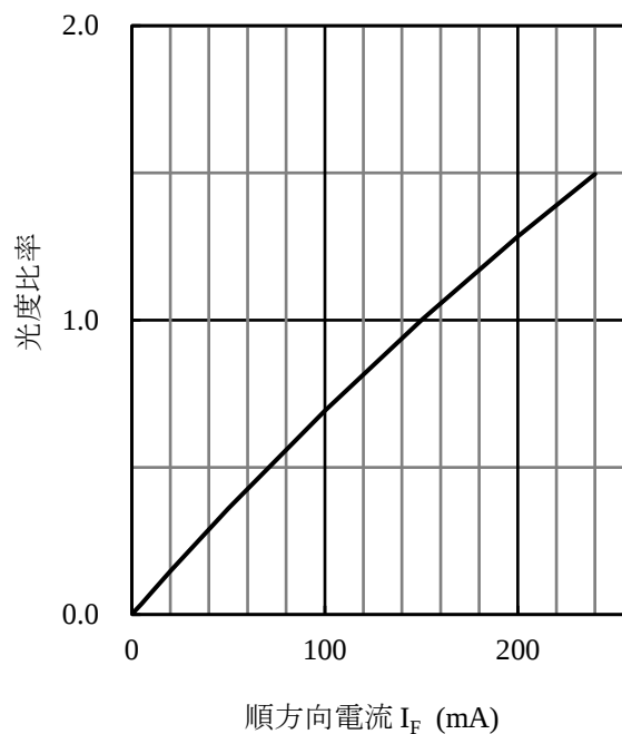
図4 光度比率 - I_F 特性
