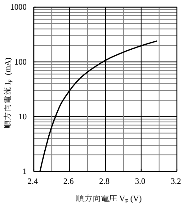
図3 I_F - V_F 特性
