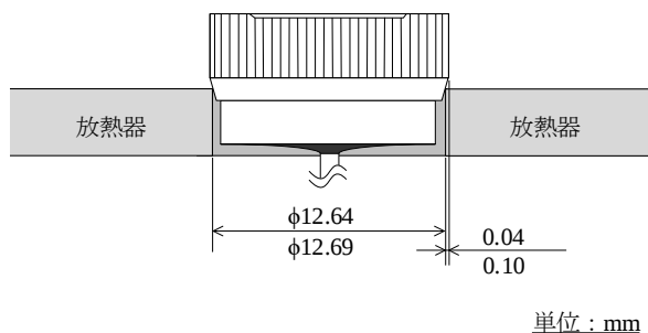
図 7 推奨穴サイズと圧入代
