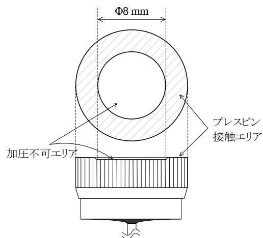
図 8 プレスピン接触エリア
