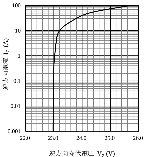
図5 I_Z - V_Z 代表特性
