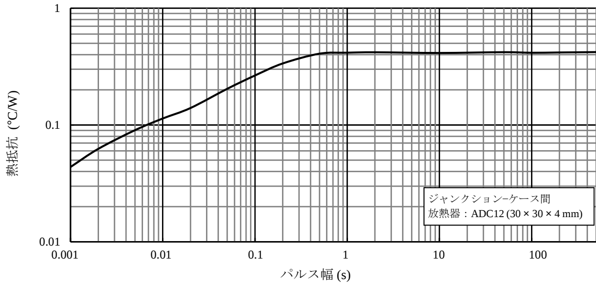
図 6 代表過渡熱抵抗特性 (2)
