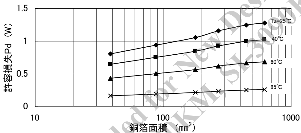
銅箔面積—許容損失 T_{j\max}=100^{\circ}\text{C}
