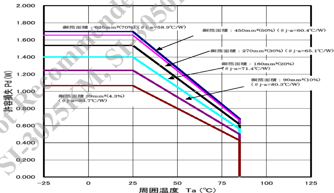
SI-3000KMシリーズ熱減定格曲線
