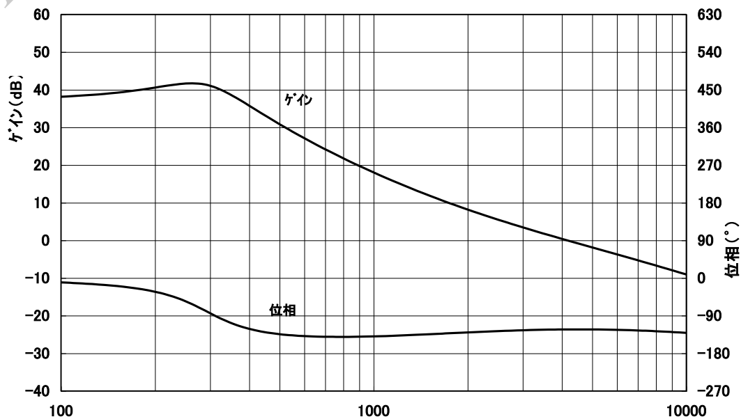
チョッパーReg ゲイン、位相特性例
