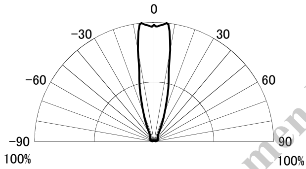
指向特性图
