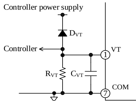
図 12-12 VT 端子周辺回路
