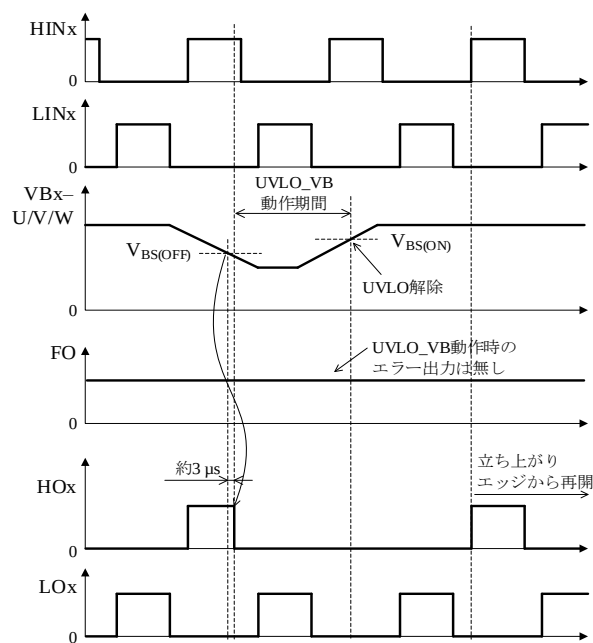
図 12-14 UVLO_VB 動作波形
