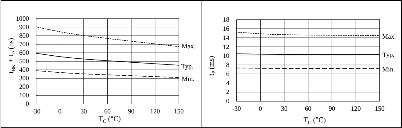
図 15-19 過電流保護ブランキング時間 t_{BK(OC)} + 内部遅延時間 t_{D(OC)} 温度特性
