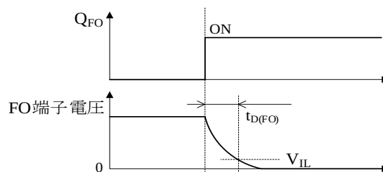
図 12-9 FO 端子の遅延時間 t_{D(FO)}
