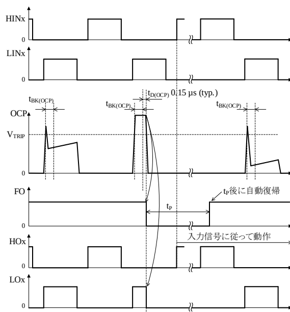
図 12-17 OCP 動作波形
