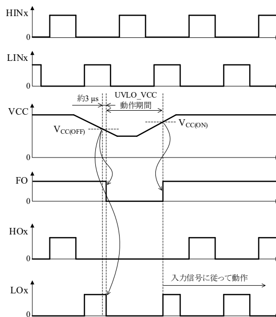
図 12-15 UVLO_VCC 動作波形
