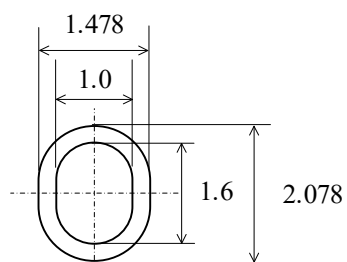
1ピン～20ピン
