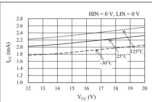
図 15-2 V_{CC} 端子電圧 V_{CC} - 制御電源電流 (3 相) I_{CC} 特性
