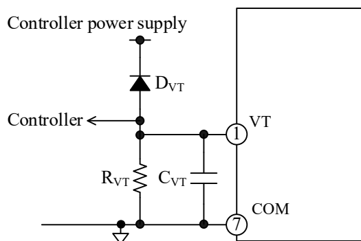
図 12-12 VT 端子周辺回路
