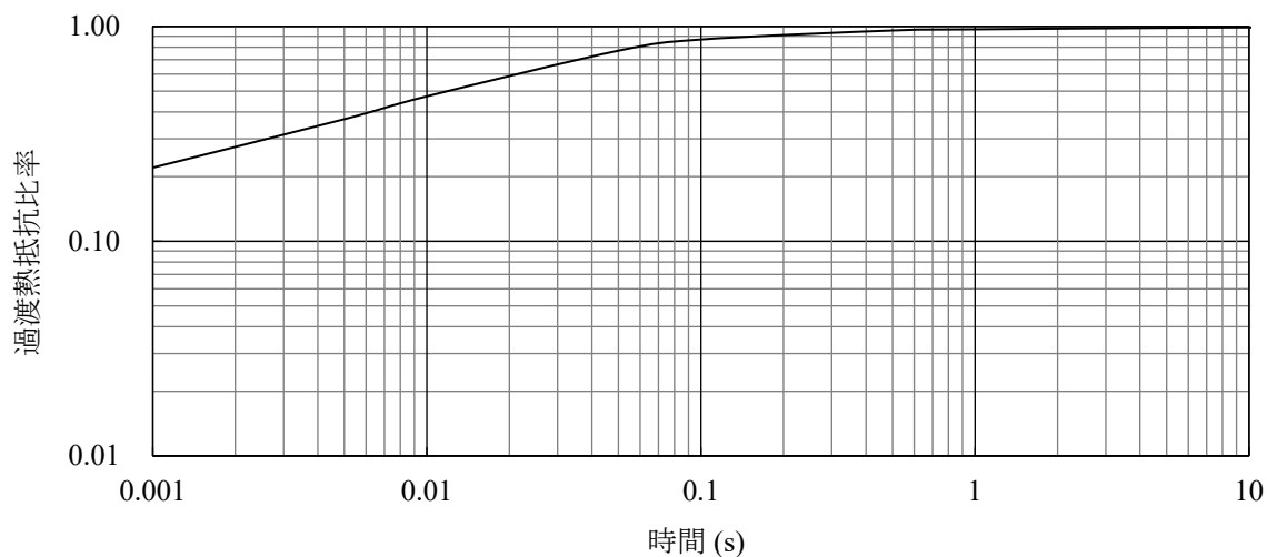
図 15-27 過渡熱抵抗比率
