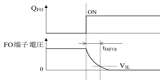
図 12-9 FO 端子の遅延時間 t_{D(FO)}
