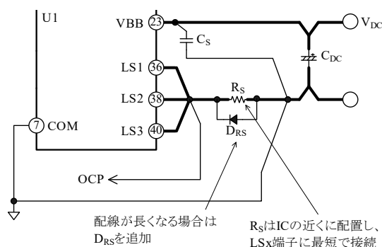
図 12-7 LSx 端子周りの配線
