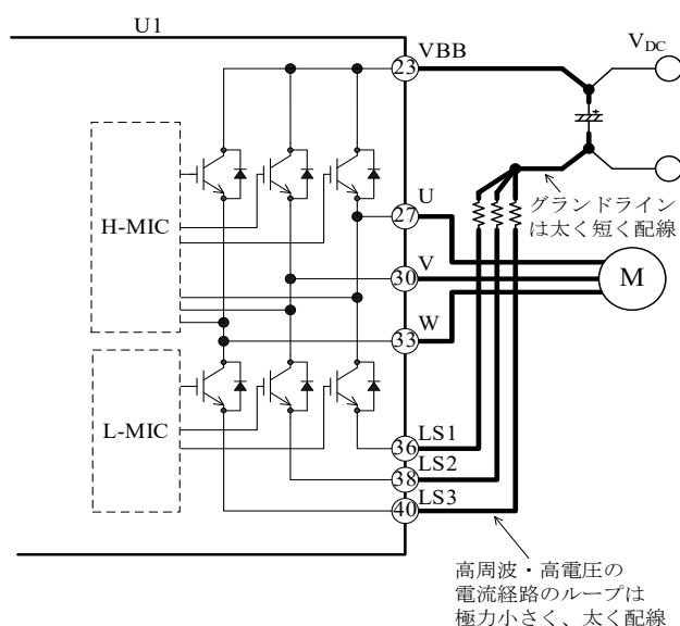
図 13-1 高周波かつ高電圧の電流経路
