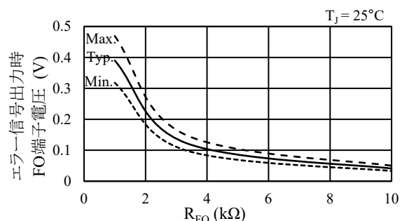
図 12-10 エラー信号出力時 FO 端子電圧 - プルアップ抵抗 R_{FO} 特性
