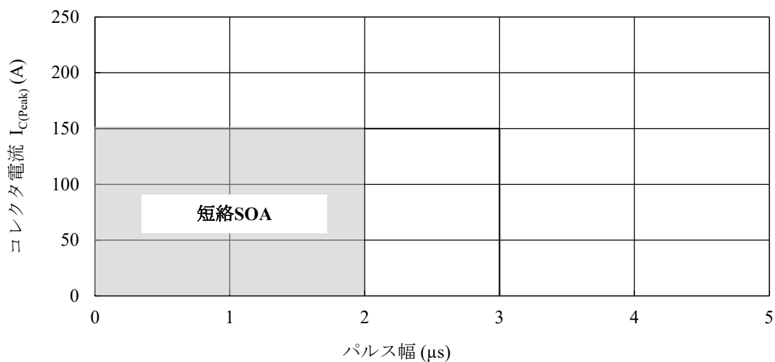
図 15-28 短絡 SOA
