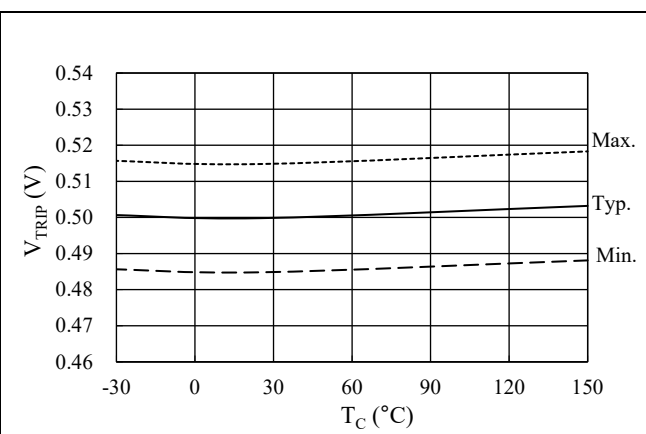
図 15-18 過電流保護動作電圧 V_{TRIP} 温度特性
