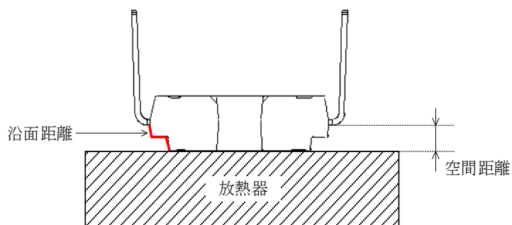
図 5-1 絶縁距離測定位置
