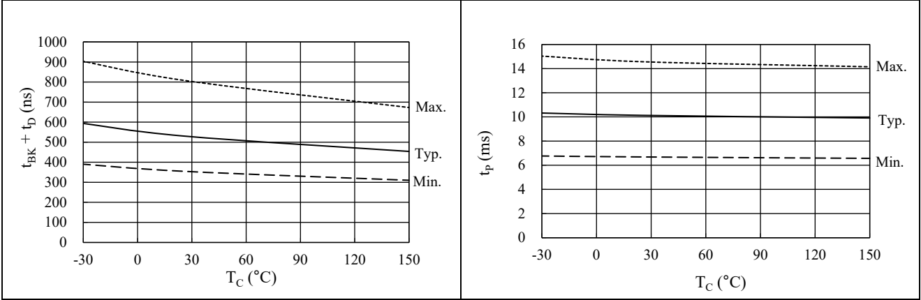
図 15-19 過電流保護ブランキング時間 t_{BK(OCP)} + 内部遅延時間 t_{D(OCP)} 温度特性
