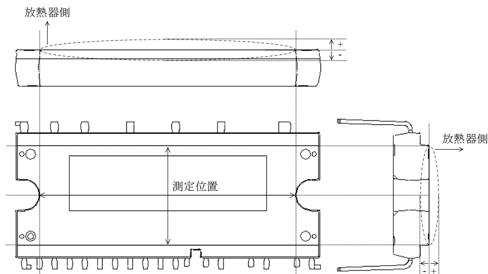
図 4-1 放熱面平坦度測定位置
