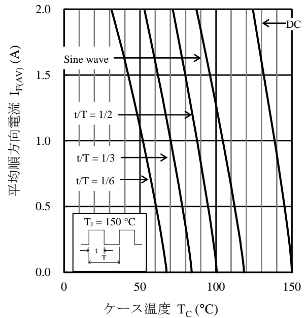
図2 I_{F(AV)} - T_C 代表特性 ( V_R = 90 V)
