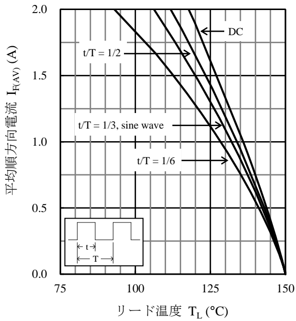
図2 I_{F(AV)} - T_L 代表特性 ( T_J = 150 °C、 V_R = 0 V)
