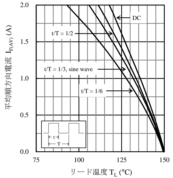
図3 I_{F(AV)} - T_L 代表特性 ( T_J = 150 °C、 V_R = 200 V)
