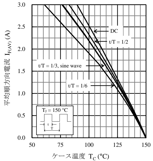
図 2 I_{F(AV)} - T_C 代表特性 ( V_R = 400 V)
