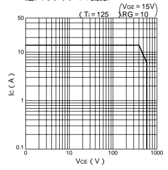
i-c-PW特性
