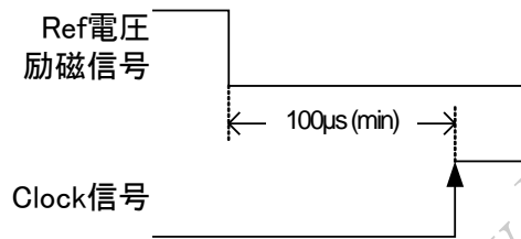
図 15-7 Disable 解除と Clock 入力のタイミング
