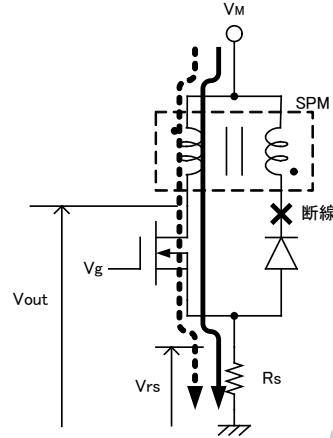
図 14-7 負荷オープン保護動作
