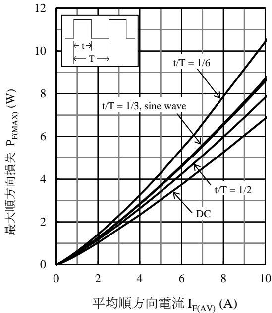
図 5 P_{F(MAX)} - I_{F(AV)} 特性 ( T_J = 150 °C)
