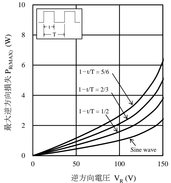
図 6 P_{R(MAX)} - V_R 特性 ( T_J = 150 °C)
