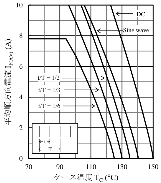
図 4 I_{F(AV)} - T_C 特性 ( T_J = 150 °C、 V_R = 150 V)
