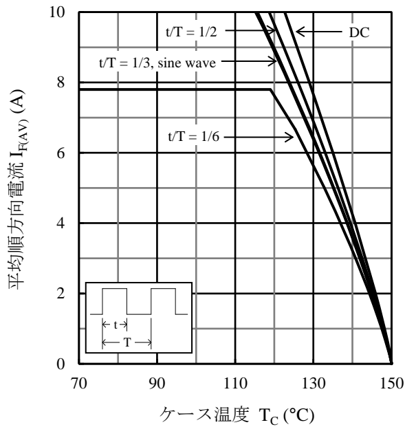
図 3 I_{F(AV)} - T_C 特性 ( T_J = 150 °C、 V_R = 0 V)
