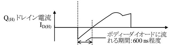
図 9-28 ZCS 確認箇所
