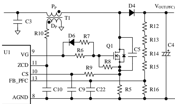
図 9-19 PFC 部回路
