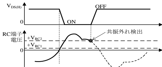
図 9-32 ハイサイド側電流共振外れ検出（重負荷時）
