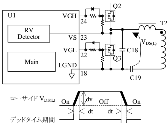
図 9-27 VS 端子とデッドタイム期間
