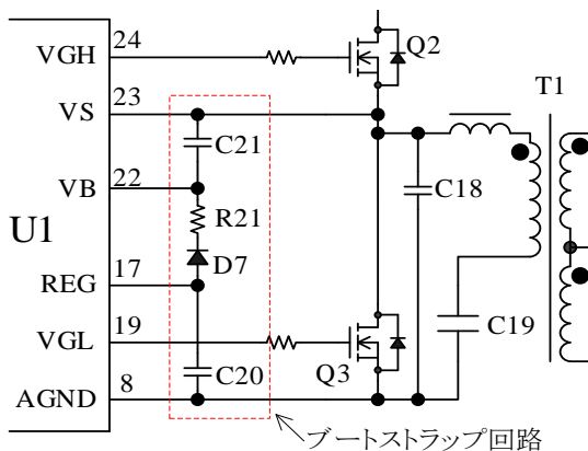
図 9-6 ブートストラップ回路
