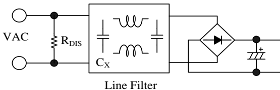
図 9-10 入力部ラインフィルタ標準回路
