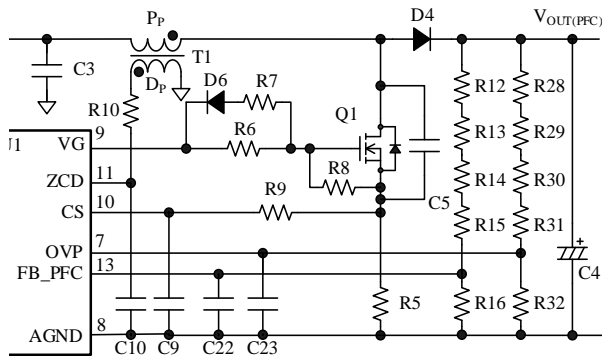
図 9-2 PFC 部回路
