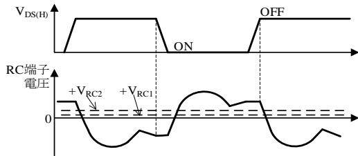
図 9-30 インダクタンス領域の RC 端子の波形
