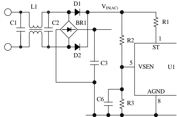
図 9-1 VSEN 端子周辺回路
