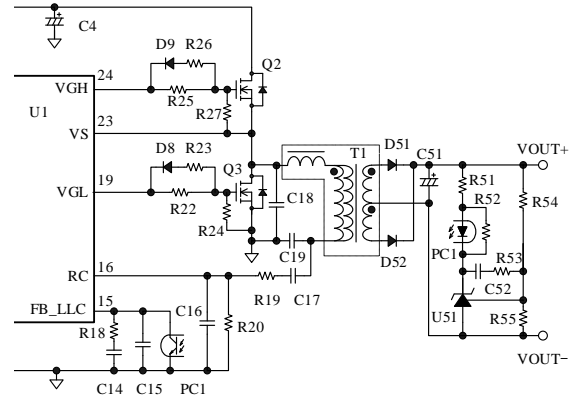
図 9-4 LLC 部回路
