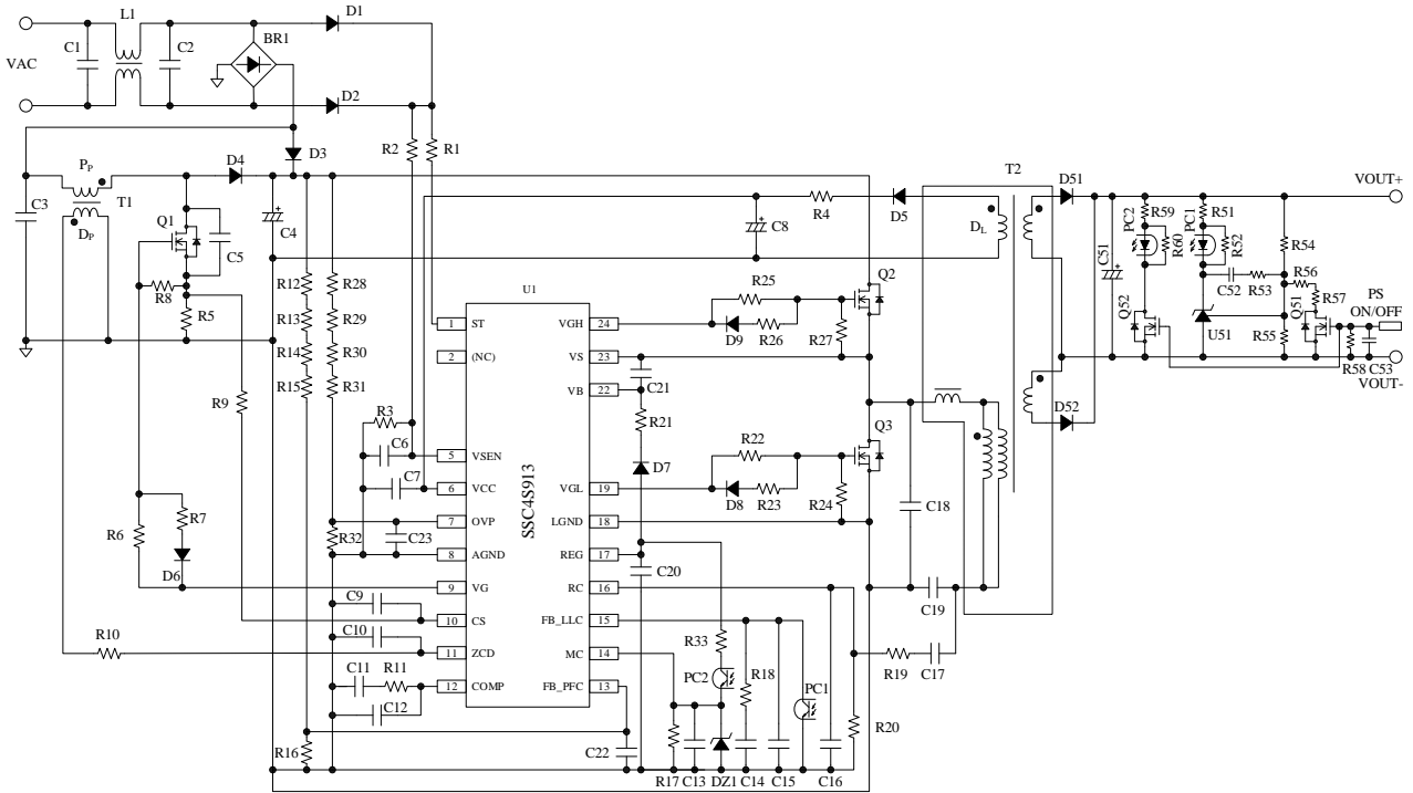
図 4-1 応用回路例
