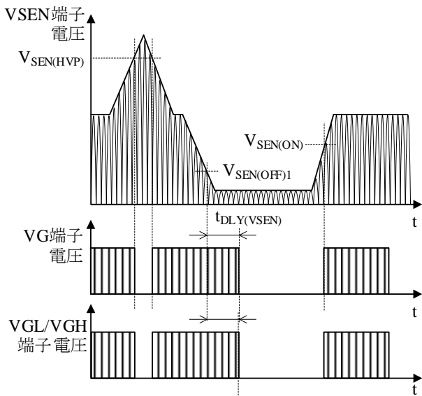
図 9-16 入力電圧保護機能動作波形
