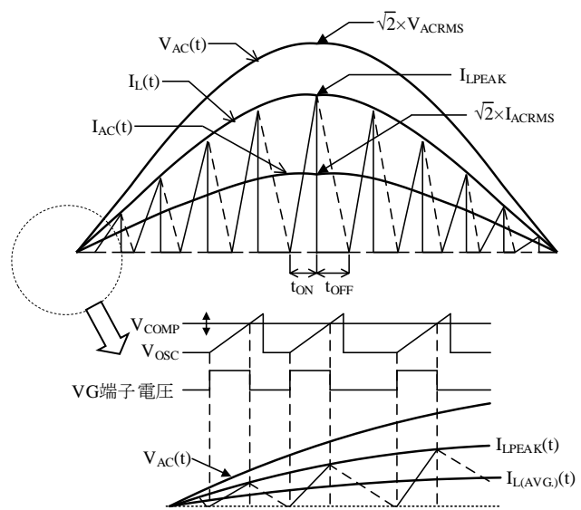
図 9-18 動作波形
