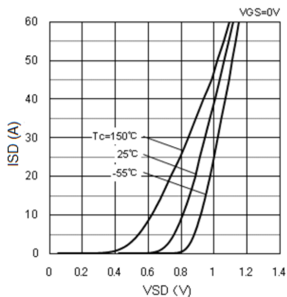
図 12 I_{SD} - V_{SD} 特性
