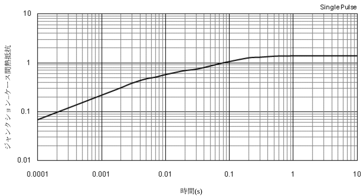
図 15 過渡熱抵抗特性
