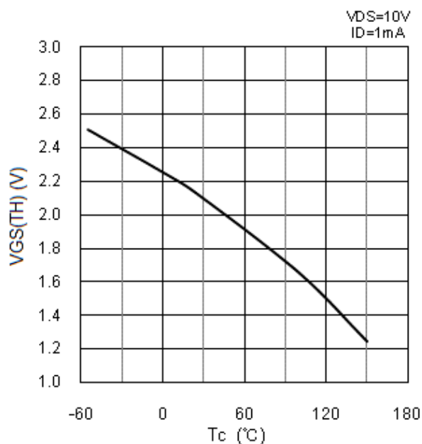
図 14 V_{GS(TH)} - T_C 特性
