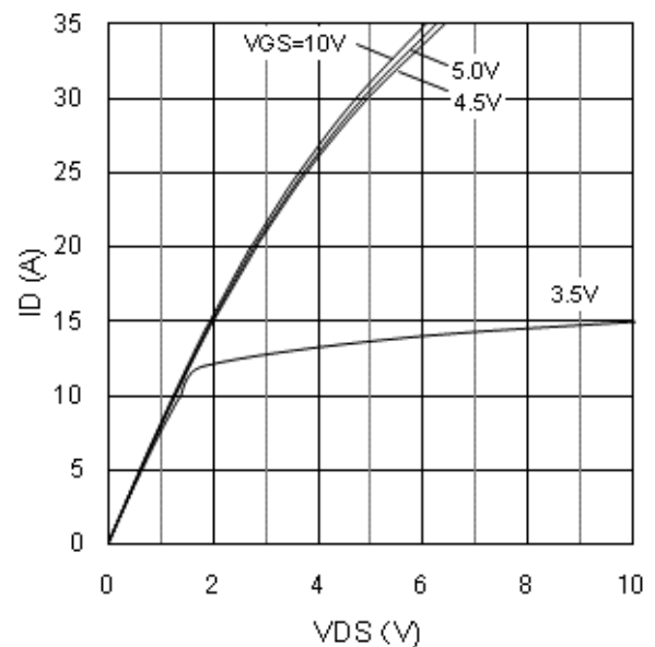
図6 I_D - V_{DS} 特性
