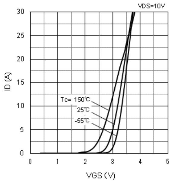
図7 I_D - V_{GS} 特性
