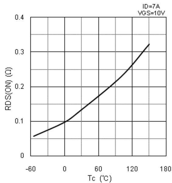
図9 R_{DS(ON)} - T_C 特性
