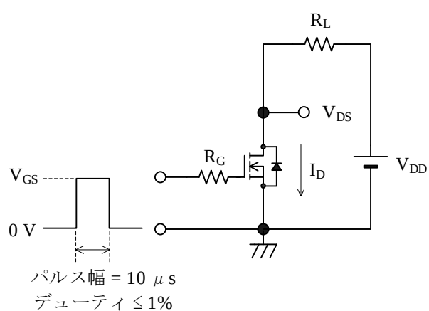
(a) 測定回路
