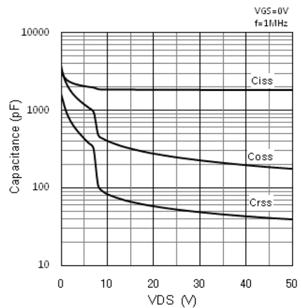
図10 容量 - V_{DS} 特性
