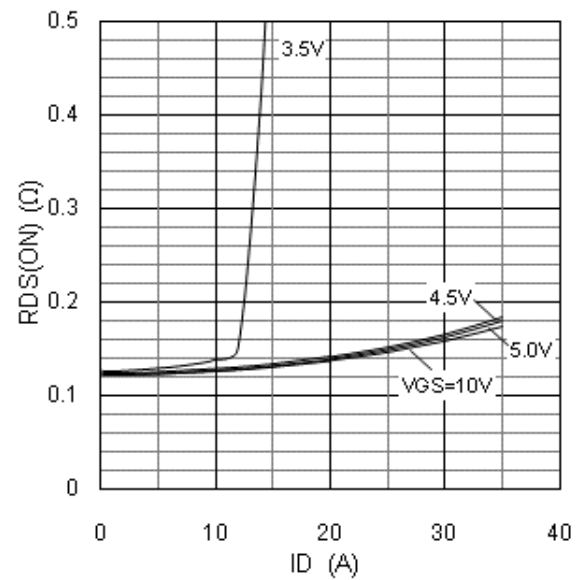
図8 R_{DS(ON)} - I_D 特性
