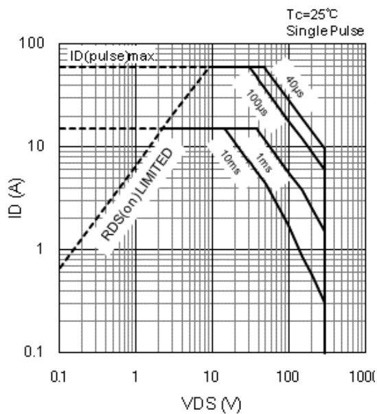
図5 安全動作領域
