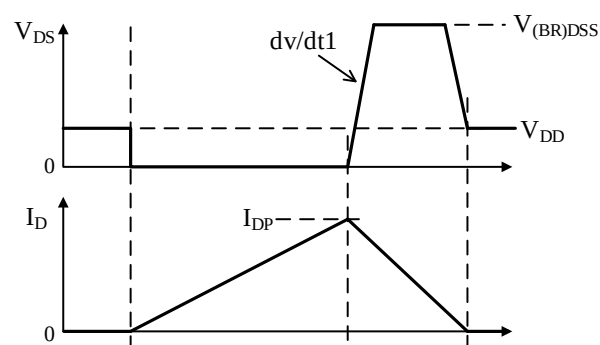
(b) スイッチング波形
