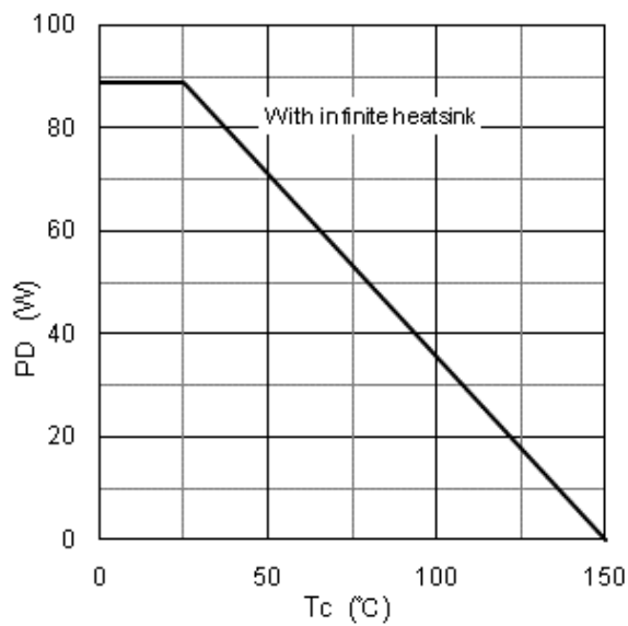
図4 P_D - T_C 特性
