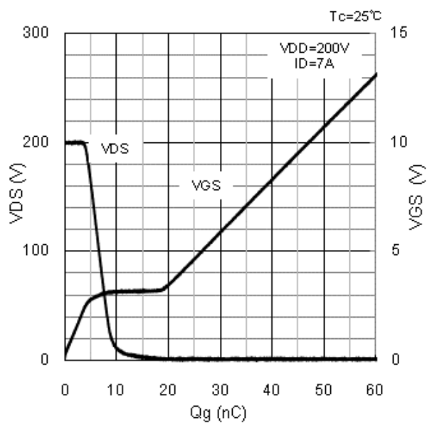
図 13 V_{DS} - Q_G 特性
