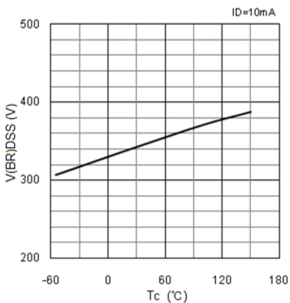
図 11 V_{(BR)DSS} - T_C 特性
