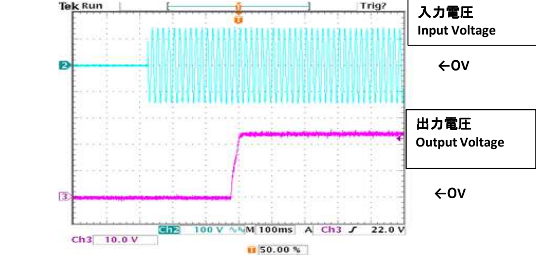
図15 出力電圧立上り波形 Fig.15 Output Voltage Rising Waveform
