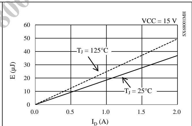
図 14-37 ローサイドスイッチング損失
