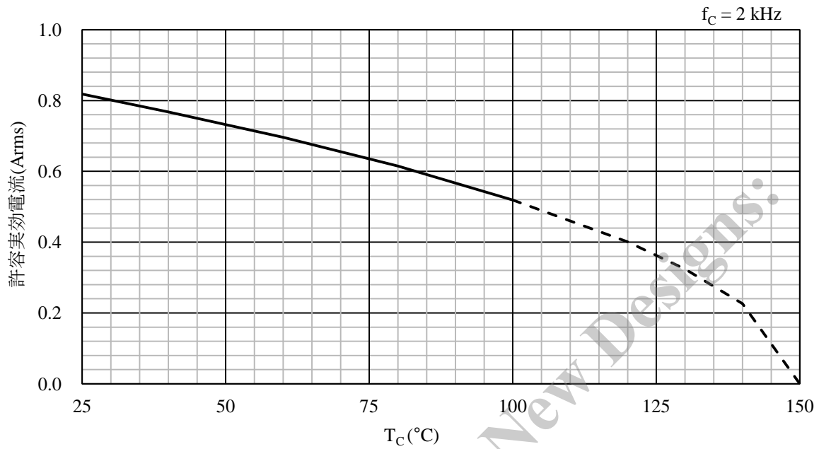
図 14-44 SX68002MH 許容電流曲線 ( f_c = 2 \text{ kHz} )
