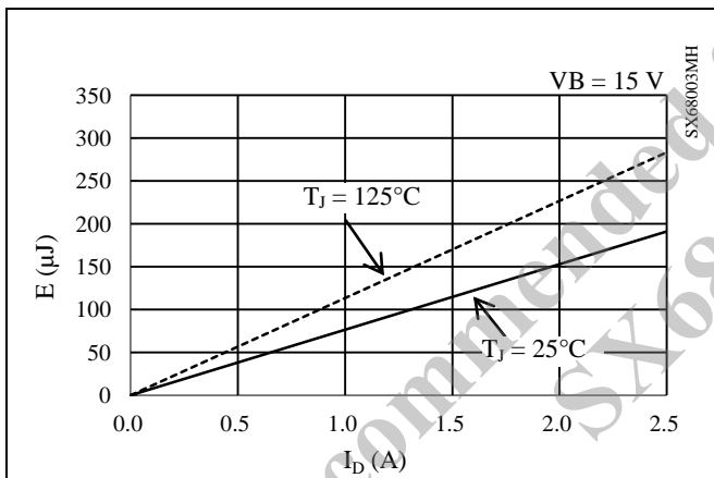
図 14-40 ハイサイドスイッチング損失
