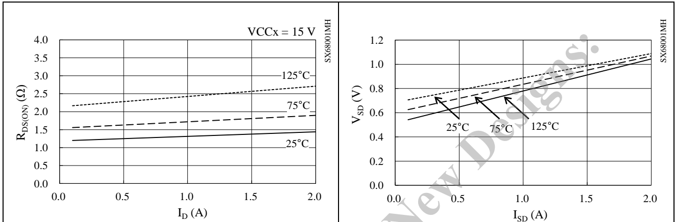
図 14-30 パワーMOSFET R_{DS(ON)} - I_D 特性
