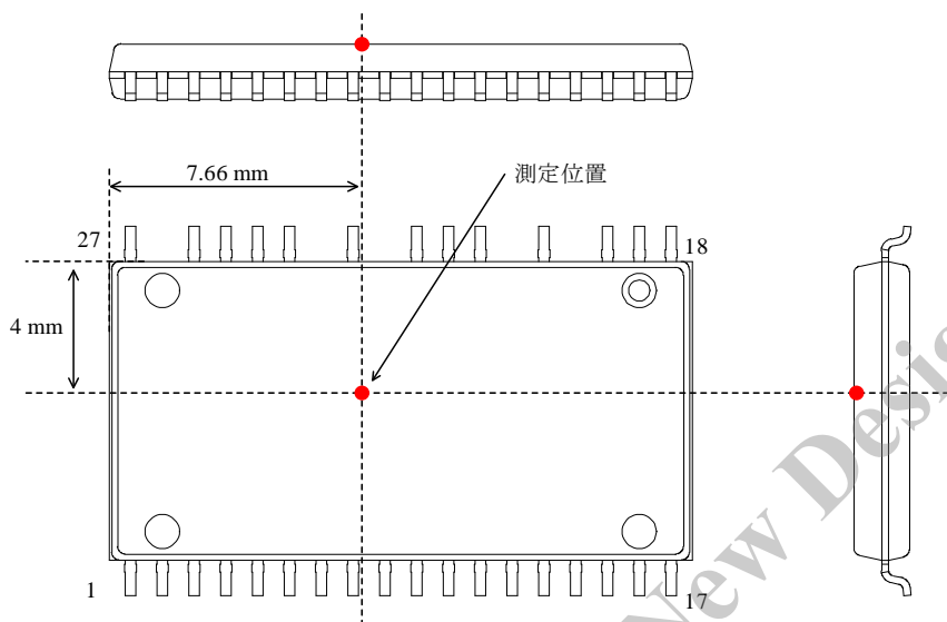
図 3-1 ケース温度測定位置
