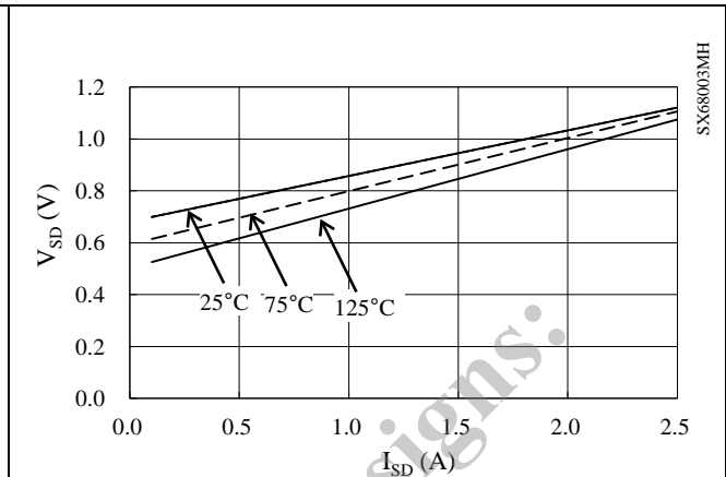
図 14-35 パワーMOSFET V_{SD} - I_{SD} 特性
