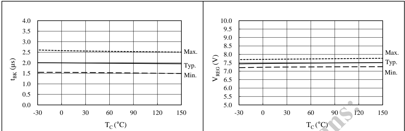
図 14-28 過電流保護ブランキング時間 t_{BK(OCP)} 、 電流リミッタブランキング時間 t_{BK(OCL)} 温度特性
