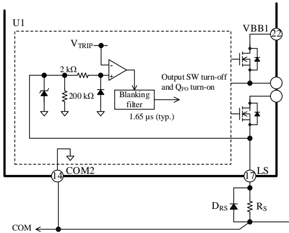
図 11-14 LS 端子の周辺回路と内部回路図
