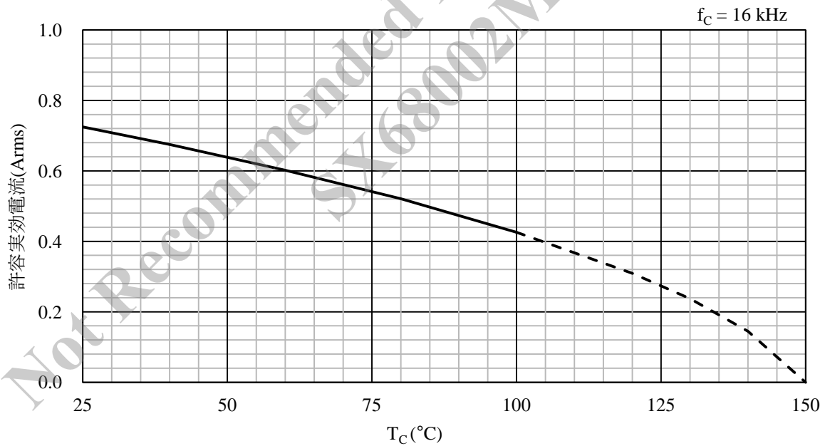
図 14-45 SX68002MH 許容電流曲線 ( f_c = 16 \text{ kHz} )
