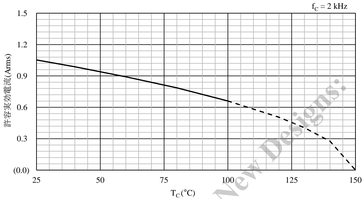
図 14-46 SX68003MH 許容電流曲線 ( f_c = 2 kHz)
