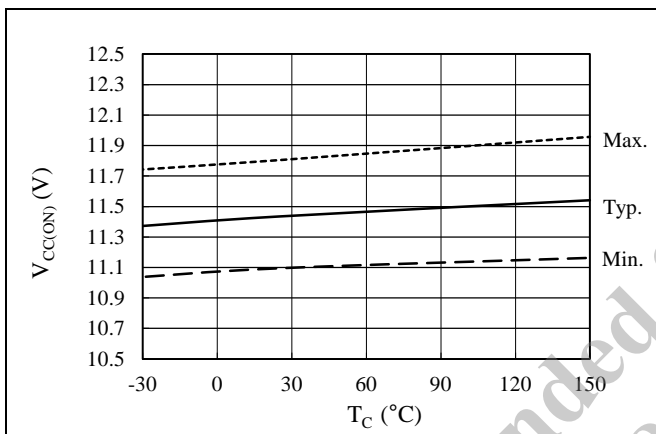
図 14-12 制御電源動作開始電圧 V_{CC(ON)} 温度特性
