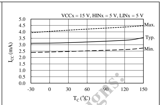
図 14-5 制御電源電流 I_{CC} 温度特性 ( I_{N_x} = 5\text{ V} )
