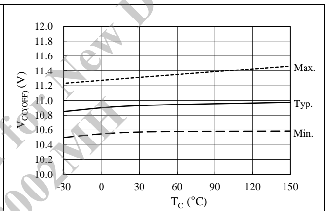
図 14-13 制御電源動作停止電圧 V_{CC(OFF)} 温度特性
