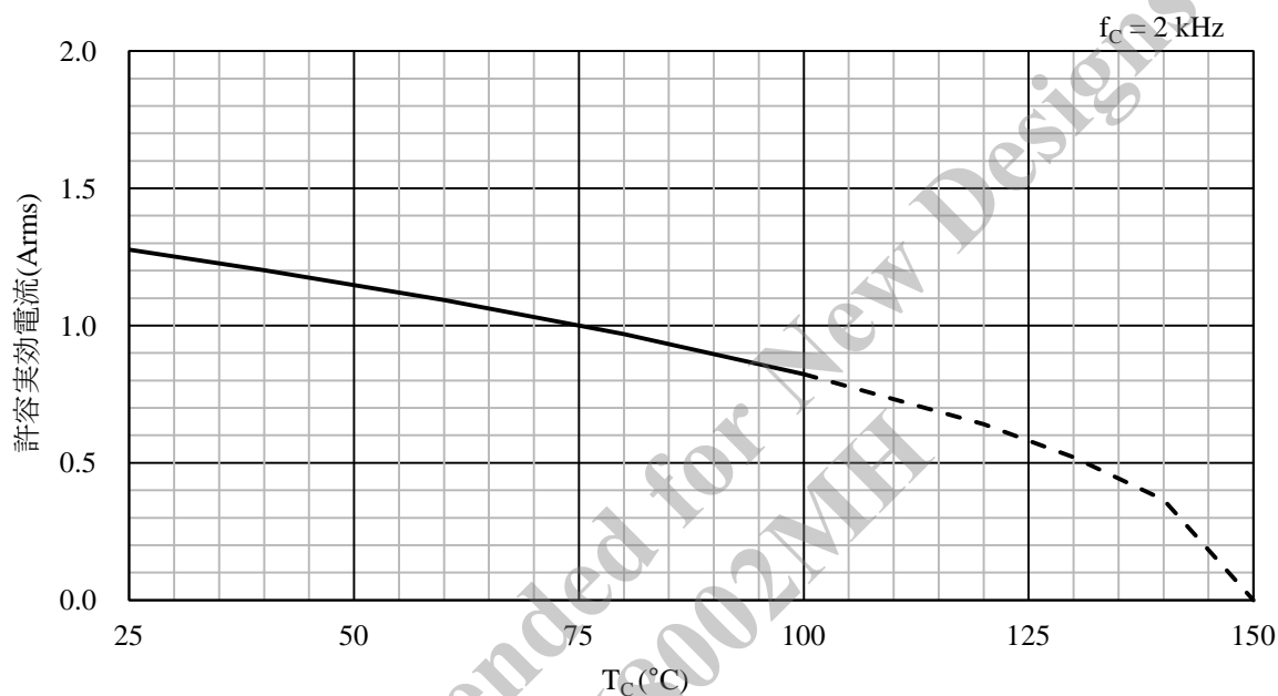
図 14-42 SX68001MH 許容電流曲線 (f c = 2 kHz)
