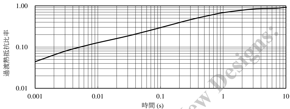
図 14-1 SX68001MH 過渡熱抵抗比率曲線
