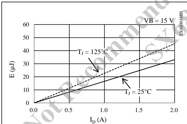
図 14-36 ハイサイドスイッチング損失
