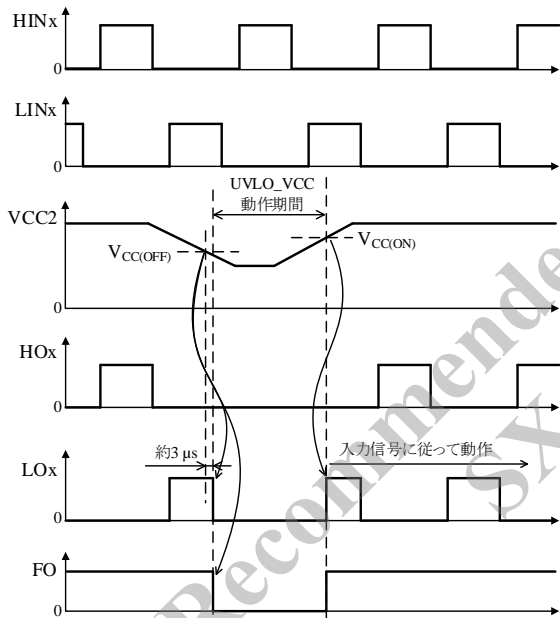
図 11-11 UVLO_VCC 動作波形
