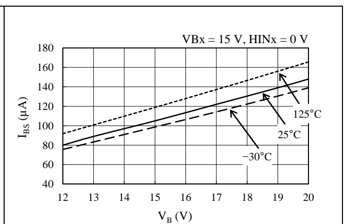
図 14-9 V_{Bx} 端子電圧 V_B - 制御電源電流 I_{BS} 特性 ( H_{IN_x} = 0\text{ V} )
