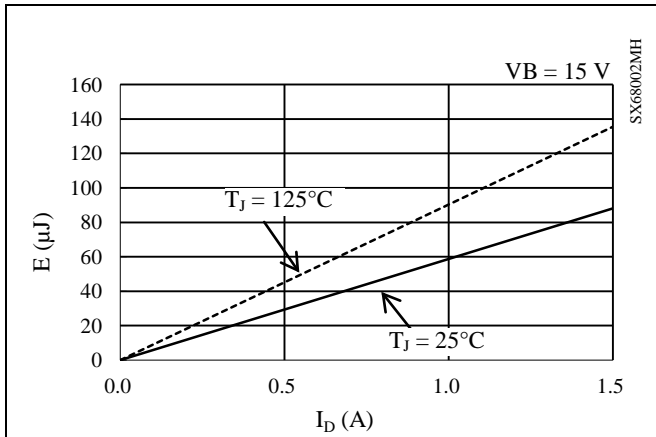
図 14-38 ハイサイドスイッチング損失
