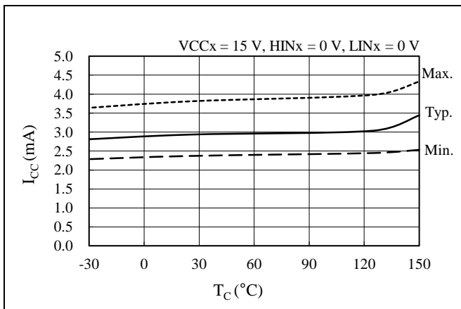
図 14-4 制御電源電流 I_{CC} 温度特性 ( I_{N_x} = 0\text{ V} )
