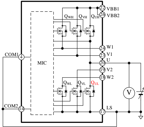
図 12-3 U相ローサイド素子(QUL)耐圧測定回路
