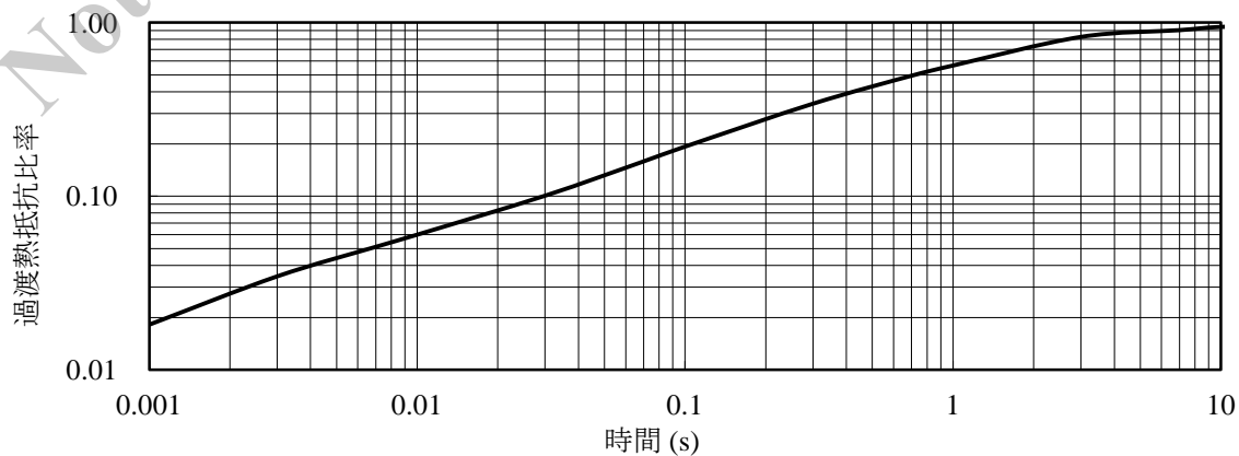
図 14-3 SX68003MH 過渡熱抵抗比率曲線
