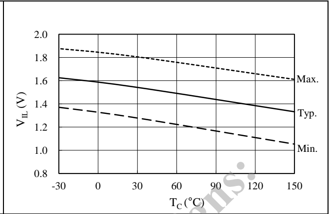
図 14-17 ローレベル入力しきい電圧 V_{IL} 温度特性
