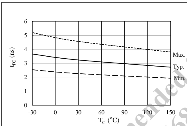
図 14-24 FO 端子フィルタ時間温度特性
