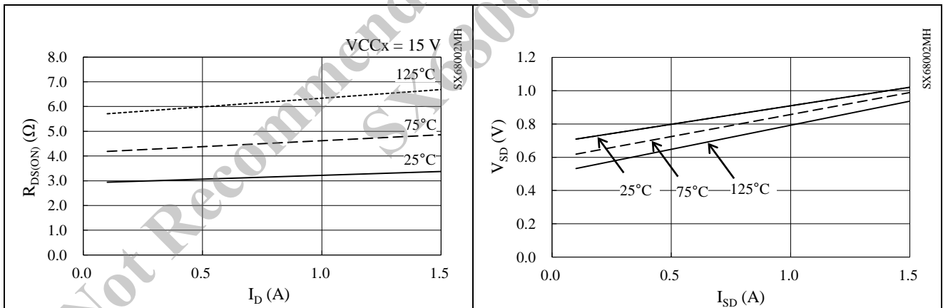
図 14-32 パワーMOSFET R_{DS(ON)} - I_D 特性
