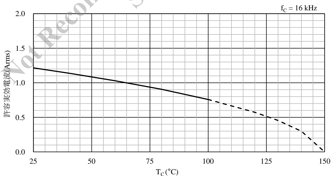
図 14-43 SX68001MH 許容電流曲線 (f c = 16 kHz)
