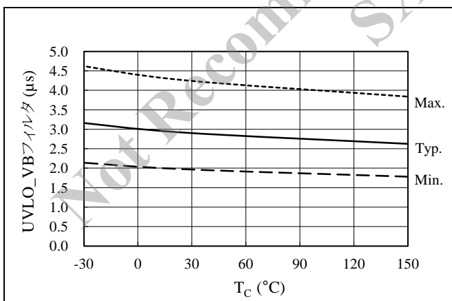
図 14-14 UVLO_VB フィルタ時間温度特性
