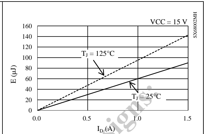
図 14-39 ローサイドスイッチング損失
