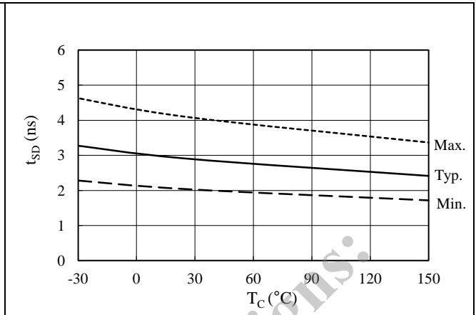
図 14-23 SD 端子フィルタ時間温度特性
