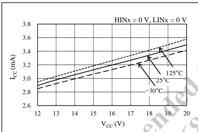
図 14-6 V_{CCx} 端子電圧 V_{CC} - 制御電源電流 I_{CC} 特性
