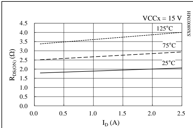
図 14-34 パワーMOSFET R_{DS(ON)} - I_D 特性
