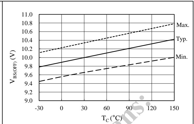
図 14-11 制御電源動作停止電圧 V_{BS(OFF)} 温度特性
