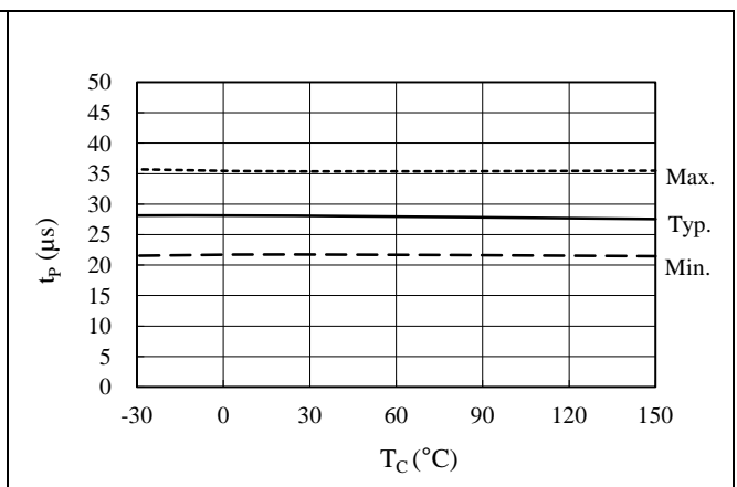
図 14-27 過電流保護保持時間 t_p 温度特性
