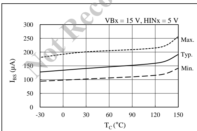
図 14-8 制御電源電流 (1 相) I_{BS} 温度特性 ( H_{IN_x} = 5\text{ V} )
