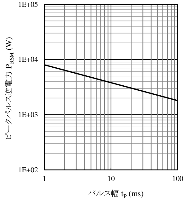
図 18 SZ-10NN40 ピークパルス逆電力 (12)
