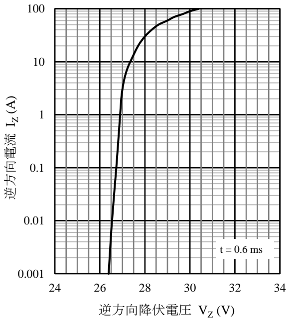
図 15 SZ-10NN27 I_Z - V_Z 代表特性
