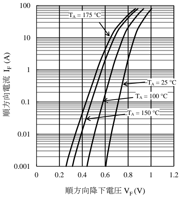
図 20 SZ-10NN40 I_F - V_F 代表特性
