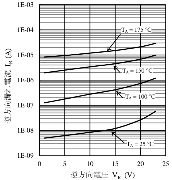
図 14 SZ-10NN27 I_R - V_R 代表特性
