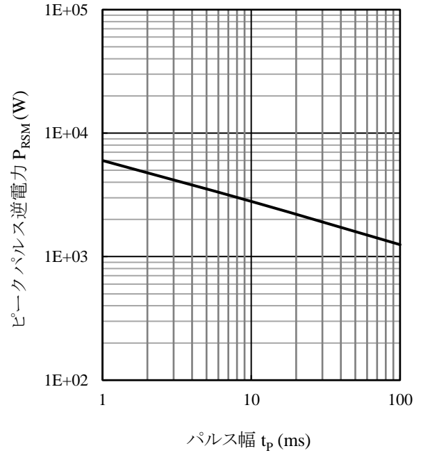
図4 SZ-10N27 ピークパルス逆電力 (6)
