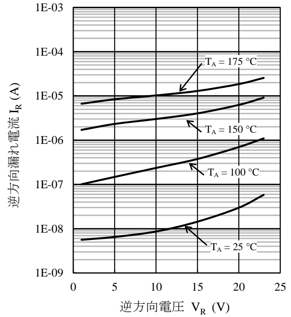
図 7 SZ-10N27 I_R - V_R 代表特性
