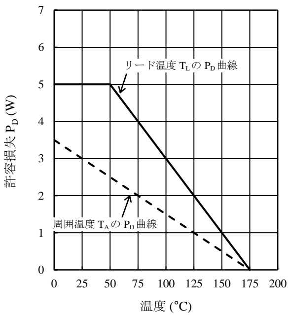
図3 SZ-10N27 許容損失曲線 (5)
