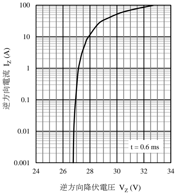
図 8 SZ-10N27 I_Z - V_Z 代表特性
