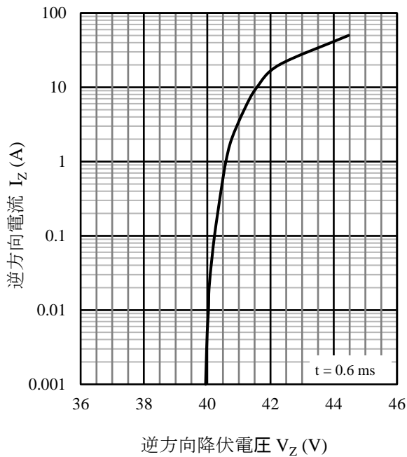
図 22 SZ-10NN40 I_Z - V_Z 代表特性
