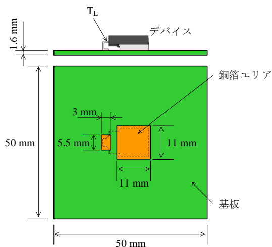
図1 リード温度測定条件
