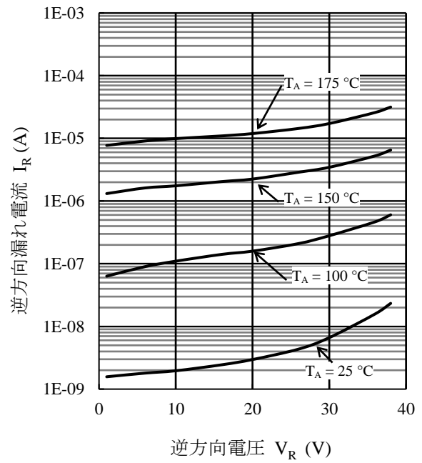
図 21 SZ-10NN40 I_R - V_R 代表特性
