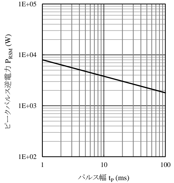
図 11 SZ-10NN27 ピークパルス逆電力 (9)
