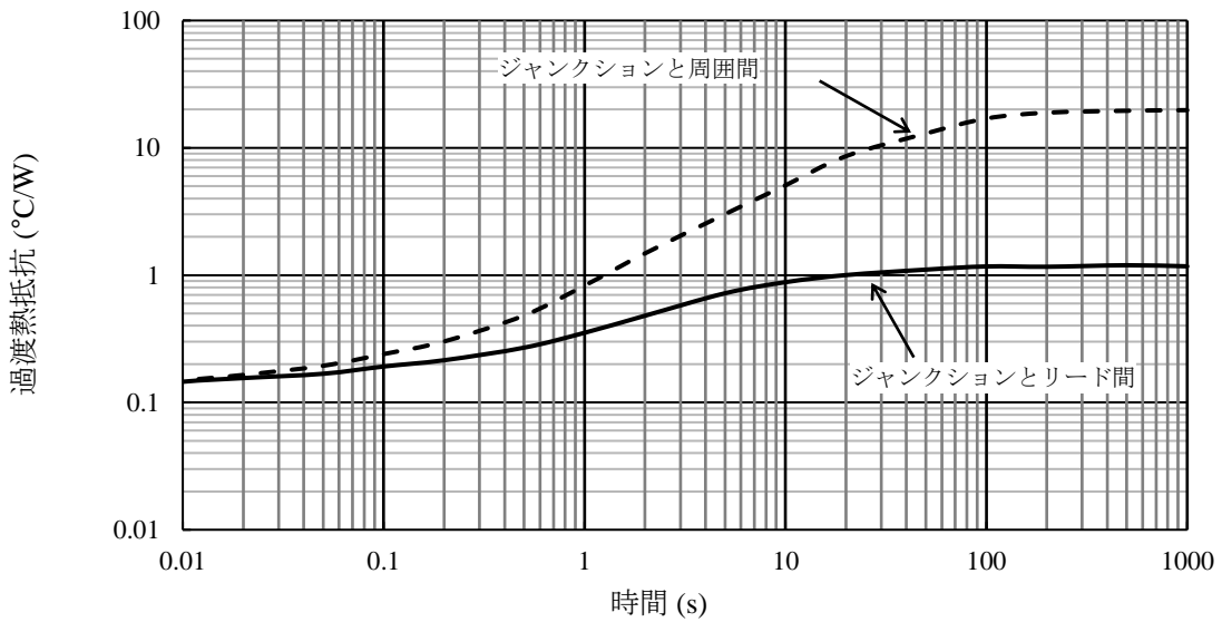
図 12 SZ-10NN27 代表過渡熱抵抗 (10)
