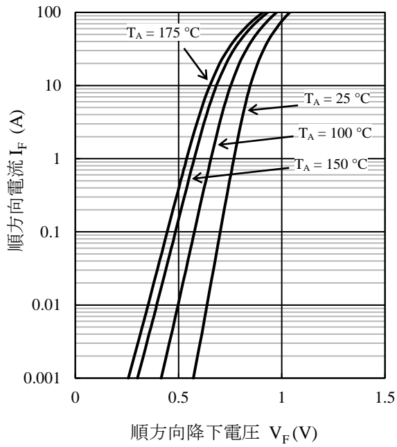
図 6 SZ-10N27 I_F - V_F 代表特性
