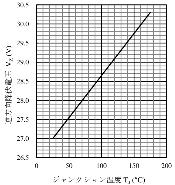
図 9 SZ-10N27 V_Z - T_J 代表特性
