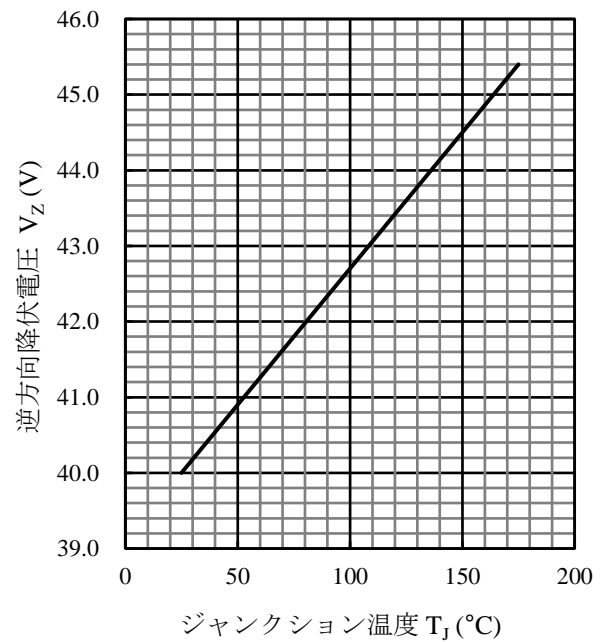
図 23 SZ-10NN40 V_Z - T_J 代表特性
