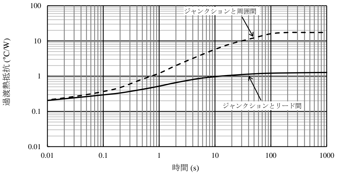
図5 SZ-10N27 代表過渡熱抵抗 (7)
