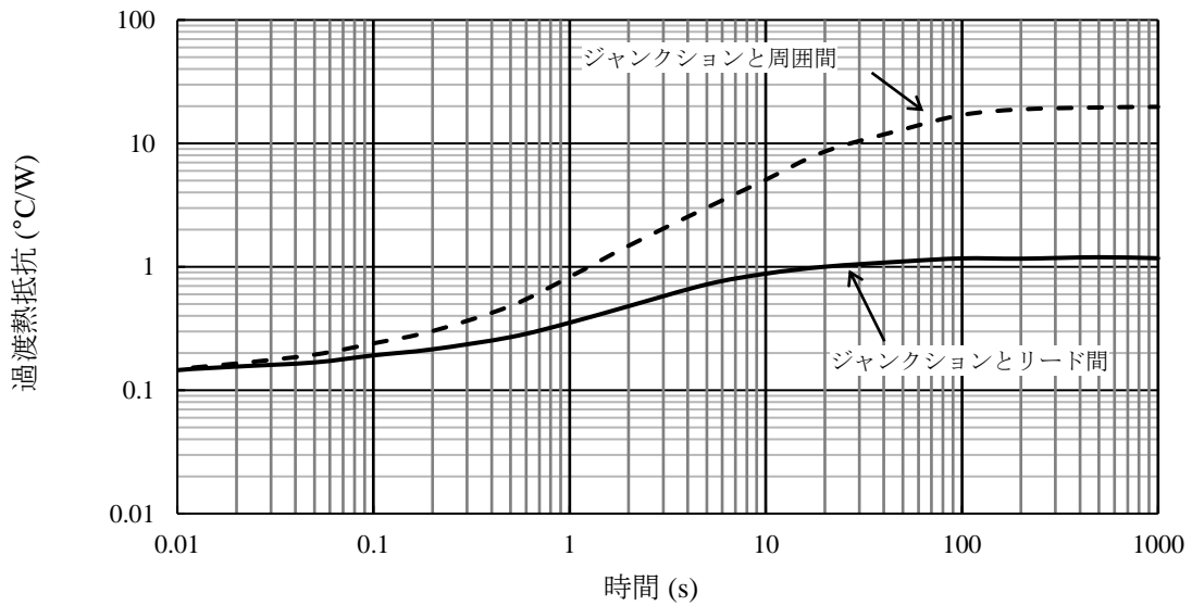
図 19 SZ-10NN40 代表過渡熱抵抗 (13)
