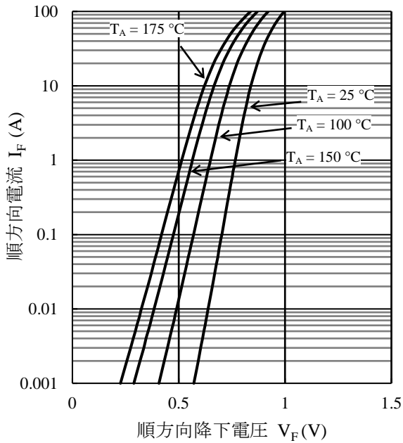
図 13 SZ-10NN27 I_F - V_F 代表特性
