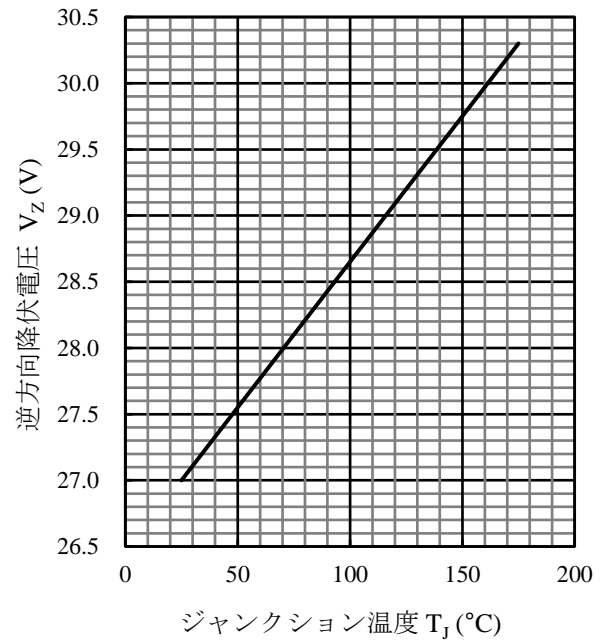
図 16 SZ-10NN27 V_Z - T_J 代表特性
