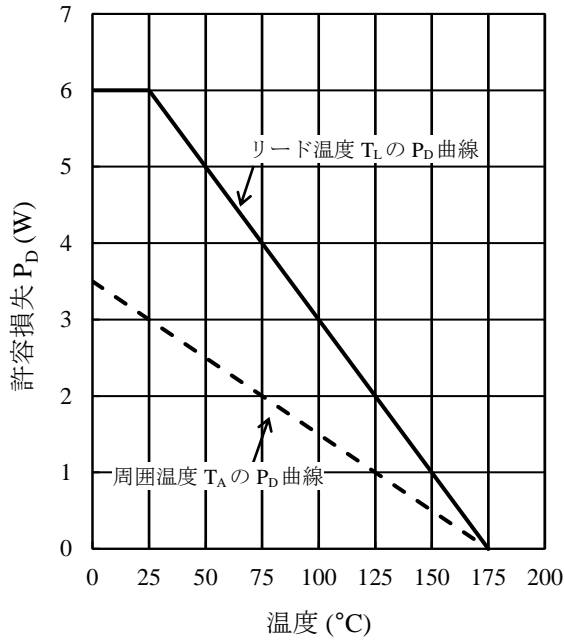
図 10 SZ-10NN27 許容損失曲線 (8)
