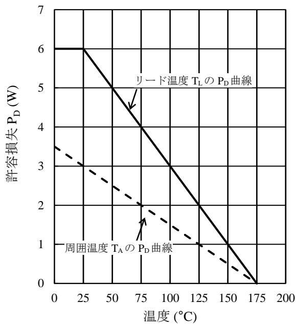
図 17 SZ-10NN40 許容損失曲線 (11)
