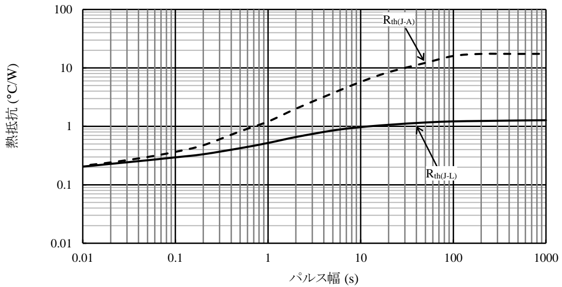
図5 SZ-10N27 代表過渡熱抵抗特性 (7)
