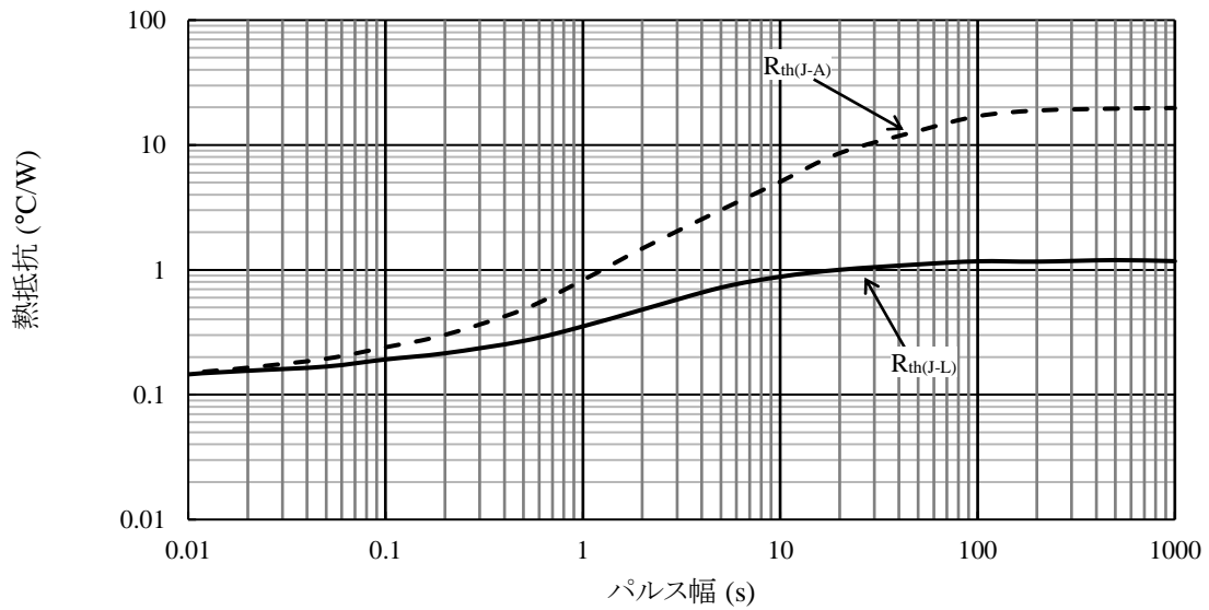
図 12 SZ-10NN27 代表過渡熱抵抗特性 (10)
