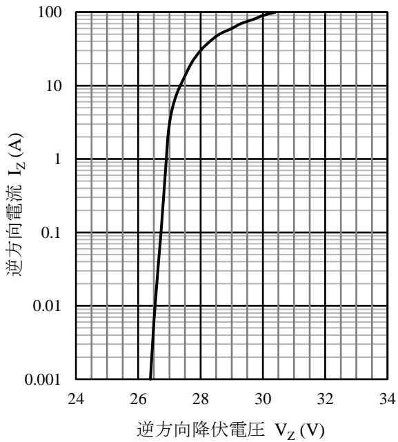
図 15 SZ-10NN27 I_Z - V_Z 代表特性 ( T_J = 25^\circ\text{C} , t = 0.6\text{ ms} )
