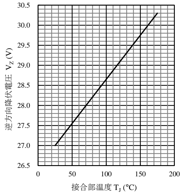
図 16 SZ-10NN27 V_Z - T_J 代表特性
