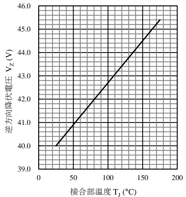
図 23 SZ-10NN40 V_Z - T_J 代表特性
