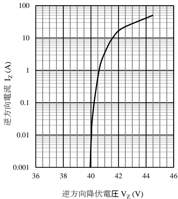
図 22 SZ-10NN40 I_Z - V_Z 代表特性 ( T_J = 25\text{ °C} , t = 0.6\text{ ms} )
