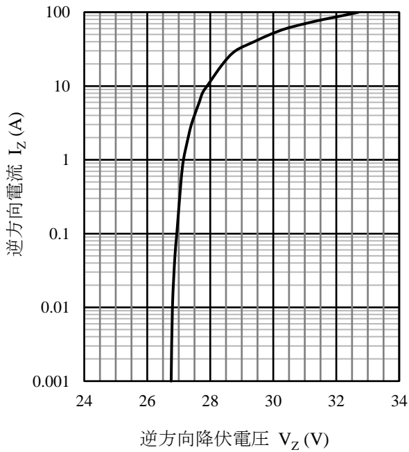
図8 SZ-10N27 I_Z - V_Z 代表特性 ( T_J = 25^\circ\text{C} , t = 0.6\text{ ms} )
