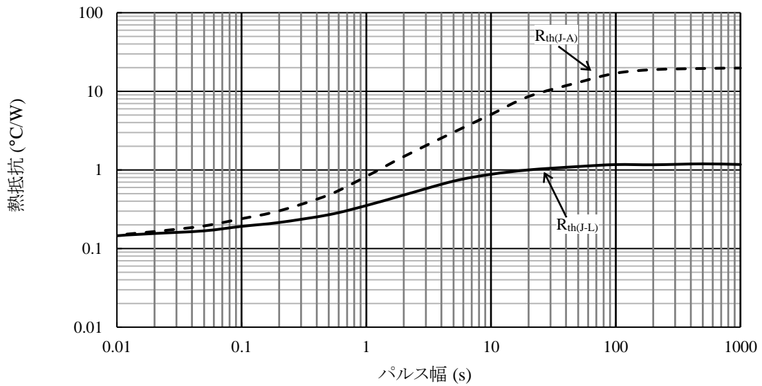
図 19 SZ-10NN40 代表過渡熱抵抗特性 (13)
