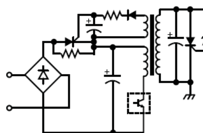
突入防止回路
